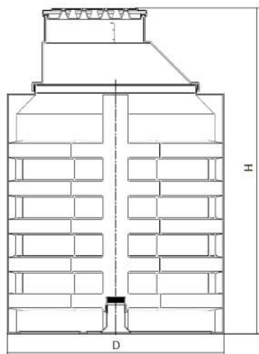
КЕССОН 3м 3
