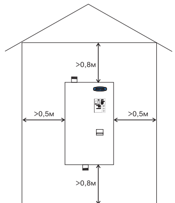
Рис. 4 Схема установки электроводонагревателя
