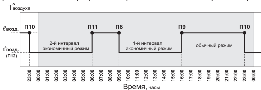
Рис. 5 График температуры воздуха в помещении для Режим 1.
