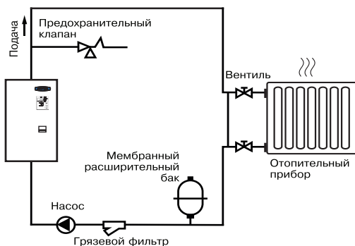
Рис. 9 Упрощенная схема подключения электроводонагревателя в отопительную систему с циркуляционным насосом
