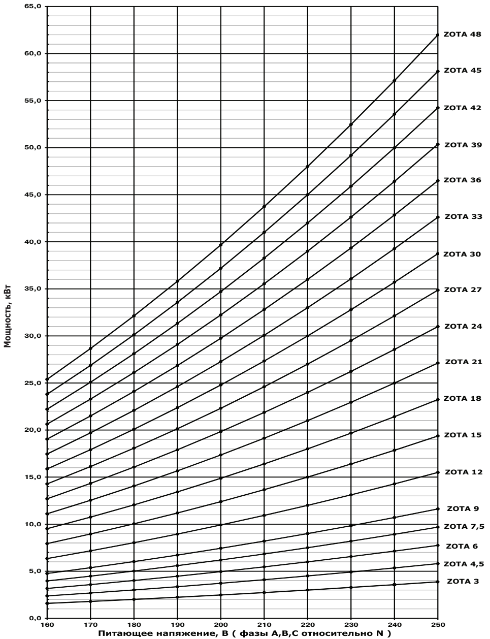
Рис. 11 График изменения мощности электроводонагревателя в зависимости от питающего напряжения
